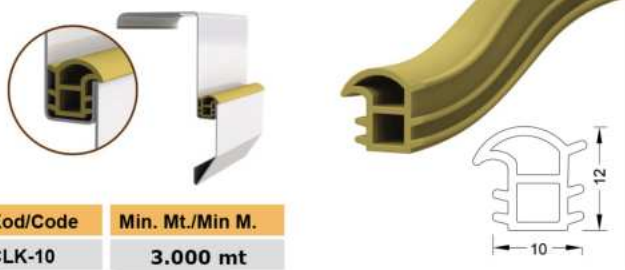
ÇELİK KAPI CONTASI Steel Door Seal
