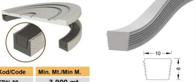
RÖGAR KAPAĞI FİTİLİ Manhole Cover Seal
