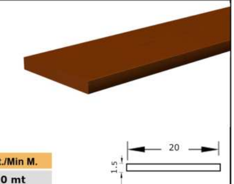
ŞERİT MIKNATIS MAGNETIC STRIP
