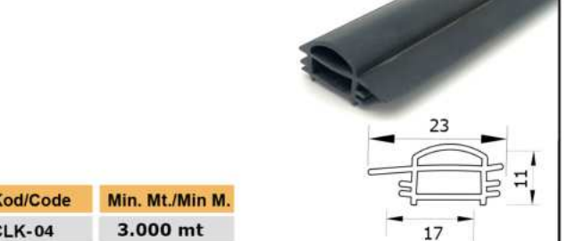
ÇELİK KAPI CONTASI Steel Door Seal
